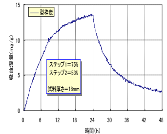
高機能無機炭の吸放湿特性
