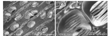
高機能炭顕微鏡写真 比表面積：300～420m 2 /g
